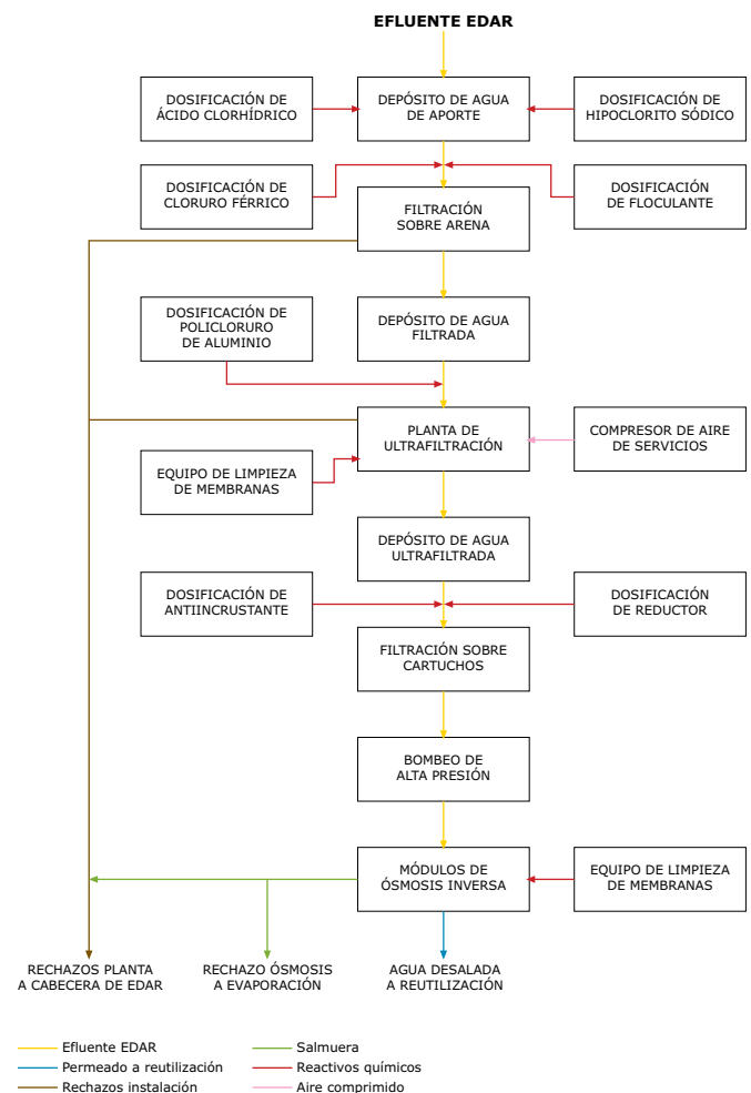
Figura 1. Diagrama de bloques de la línea de tratamiento de aguas
