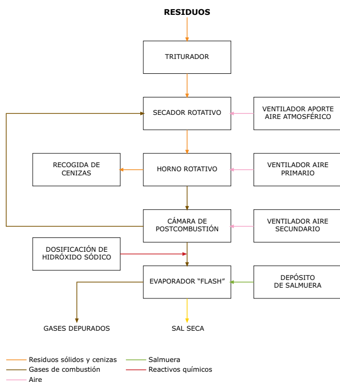
Figura 5. Diagrama de bloques de la línea de valorización energética
